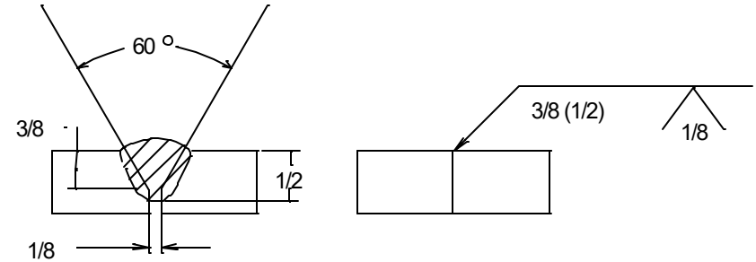
CHAMFER-GROOVE WELD
